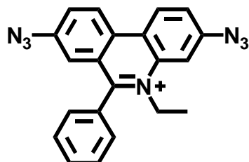
Ethidium Diazide
