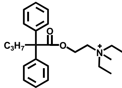
Meproadifen
