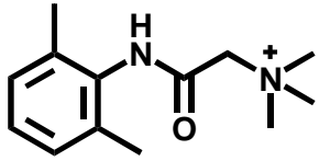
QX-222
