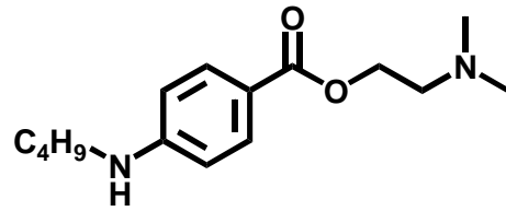
Tetracaine
